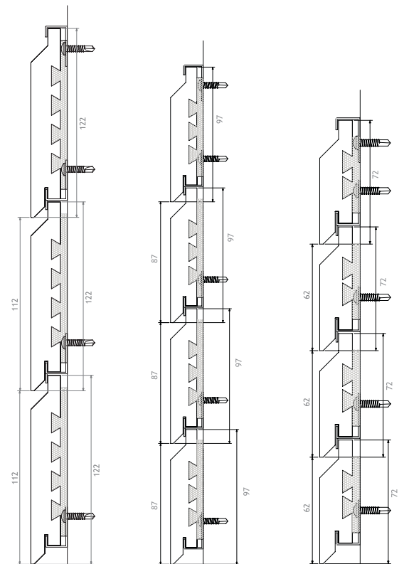
detalle de montaje
